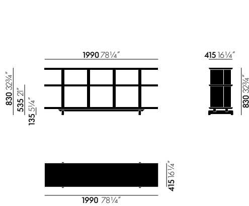
Planophore slim, 1,5 HE (hoogte-eenheden)
