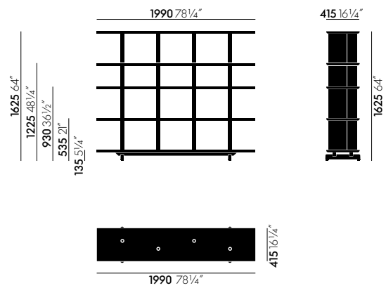
Planophore slim, 3,5 HE (hoogte-eenheden)
