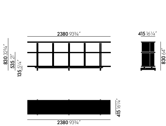
Planophore wide, 1,5 HE (hoogte-eenheden)
